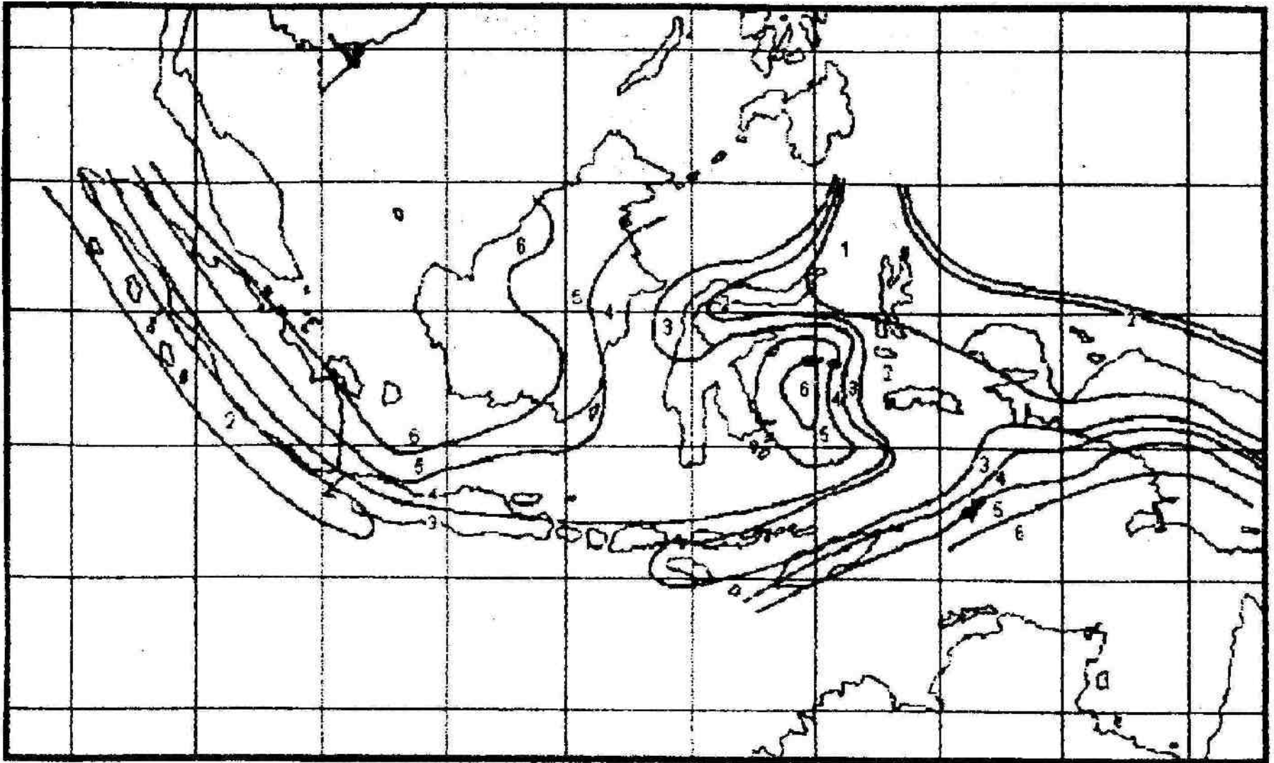
Wilayah Gempa di Indonesia (PPKGURG-1987)
